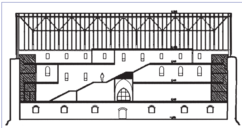
Przekrój Domu Dużego
